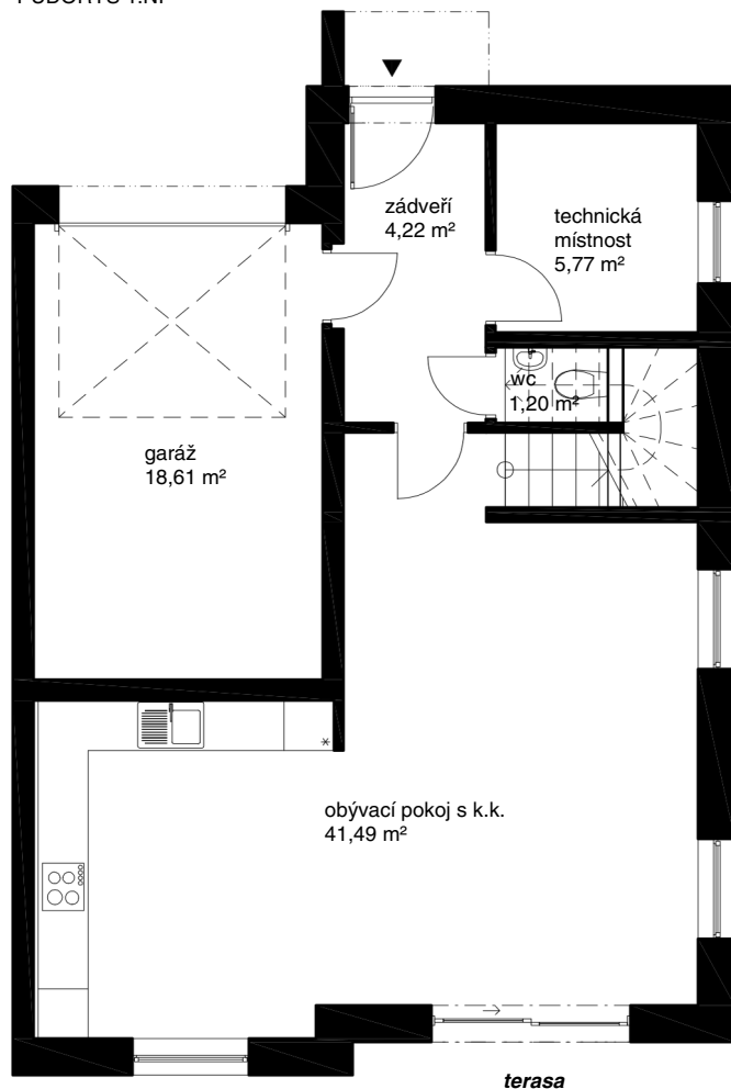
DŮM B PŮDORYS 1.NP
