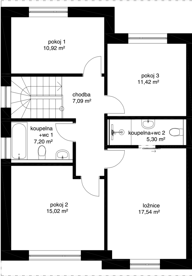
DŮM A PŮDORYS 2.NP
