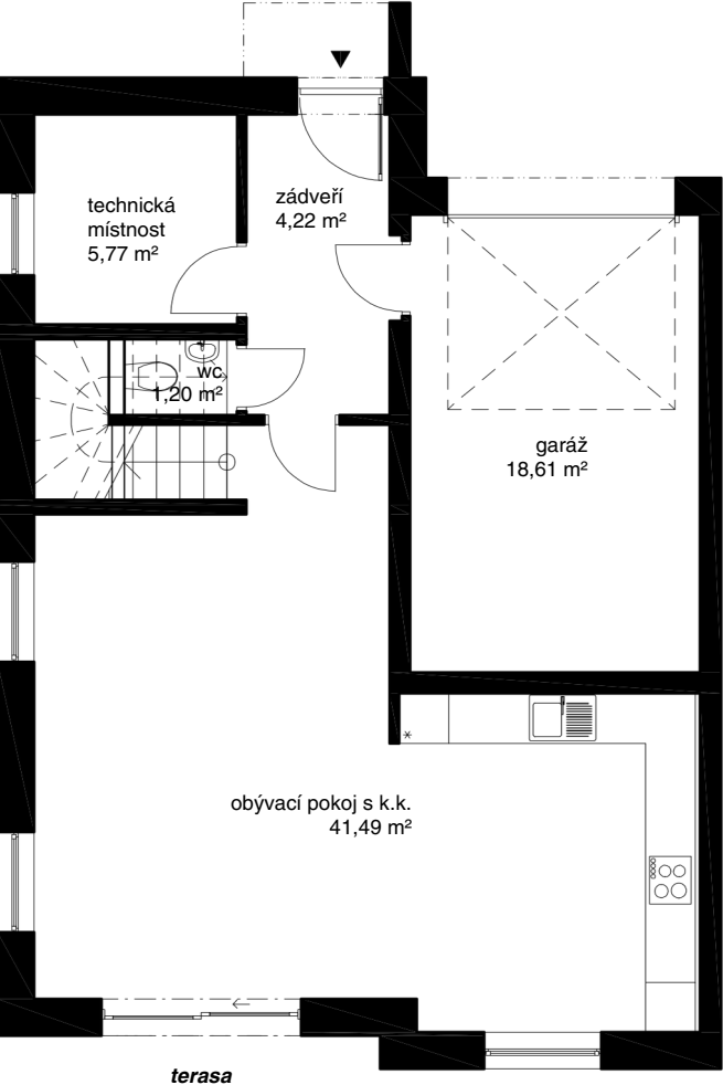
DŮM A PŮDORYS 1.NP
