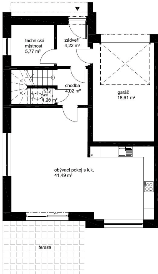
DŮM A PŮDORYS 1,NP
